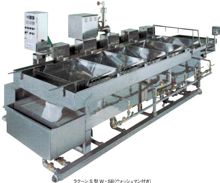
ラクーン S 型 W・5B(ウォッシュマン付き)
