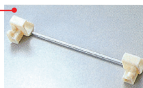
アングルクランプ(オプション) L字型またはコの字型な どの直角的に組み立て る場合に使用します。
